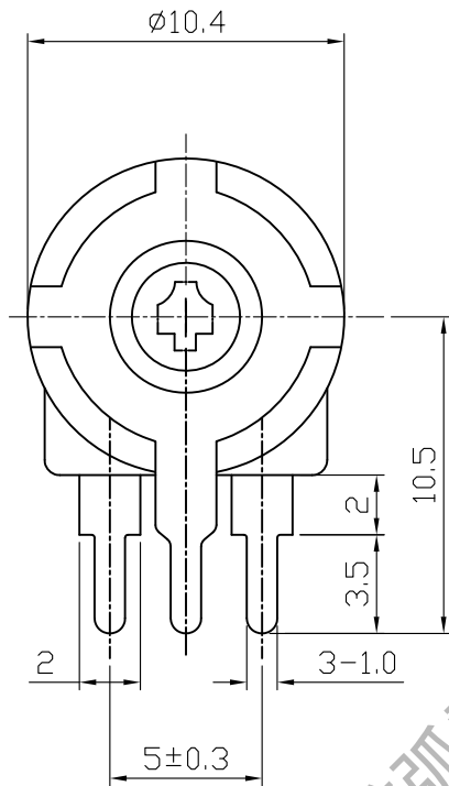
安裝孔位置圖 Mounting Hole
